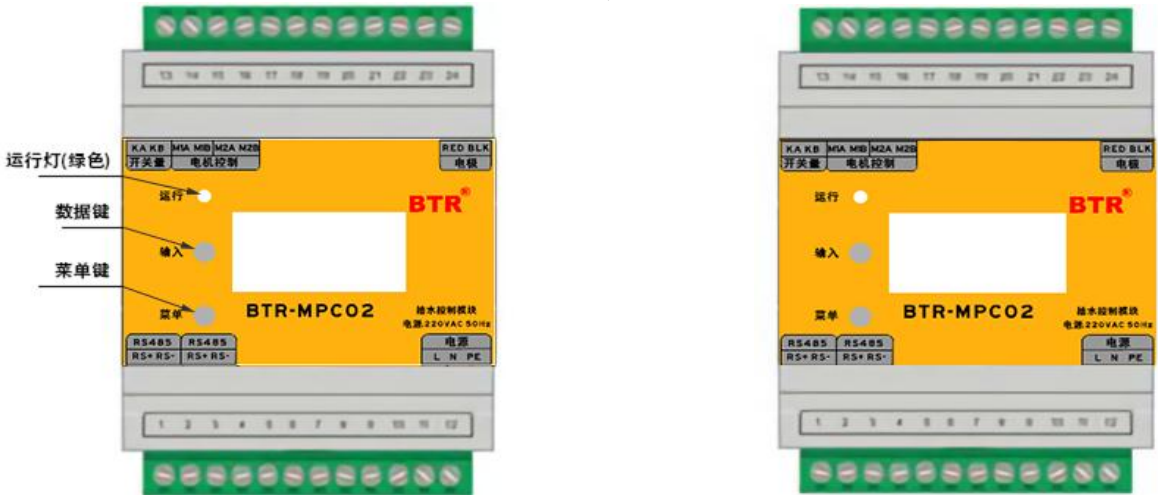
图5 标贴说明图
